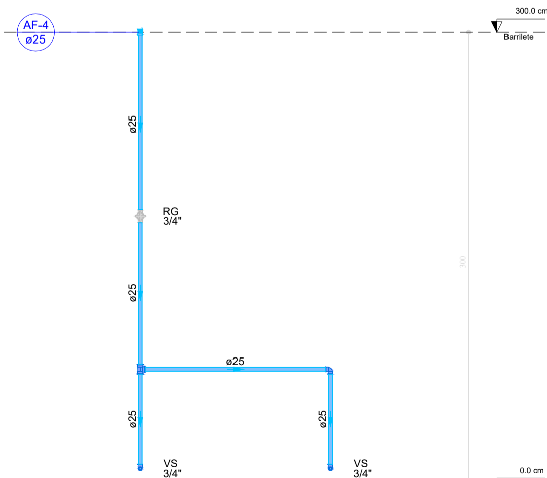
DETALHE HID-6 1:25
