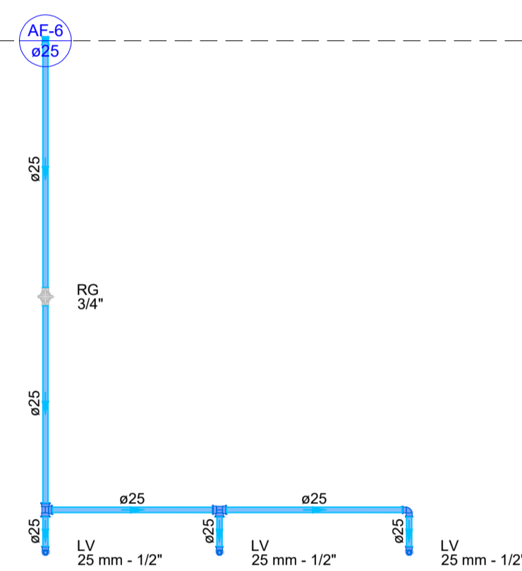
DETALHE HID-8 1:25
