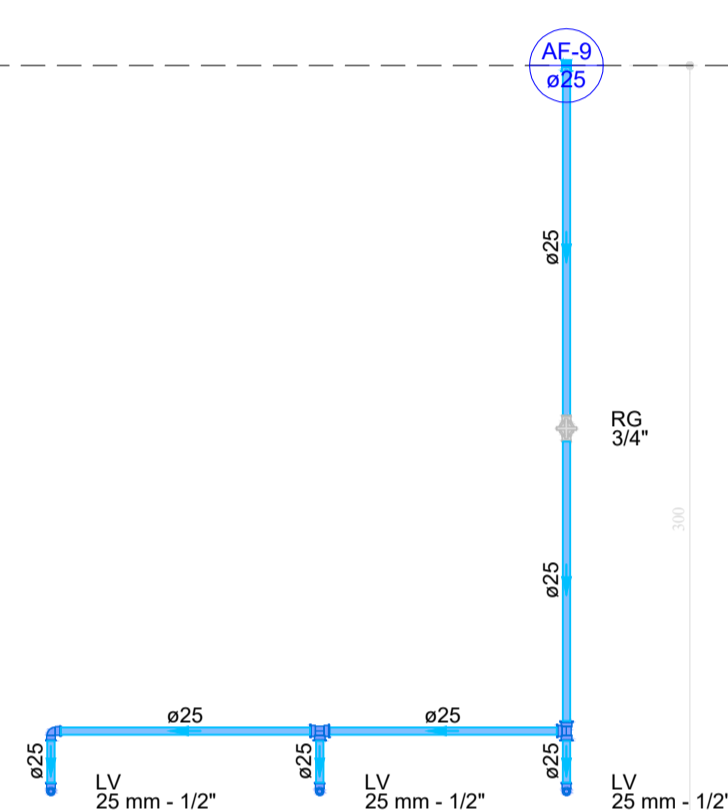
DETALHE HID-10 1:25
