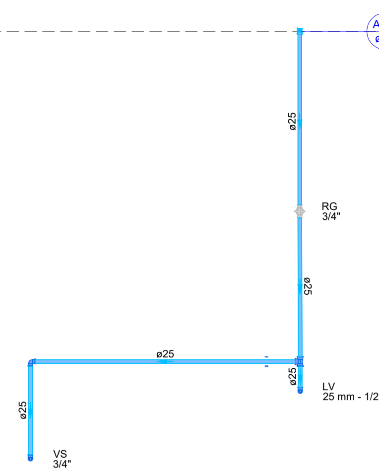
DETALHE HID-2 1:25
