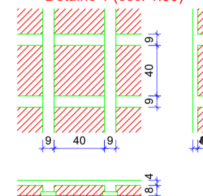
Detalhe 1 (esc. 1:30)
