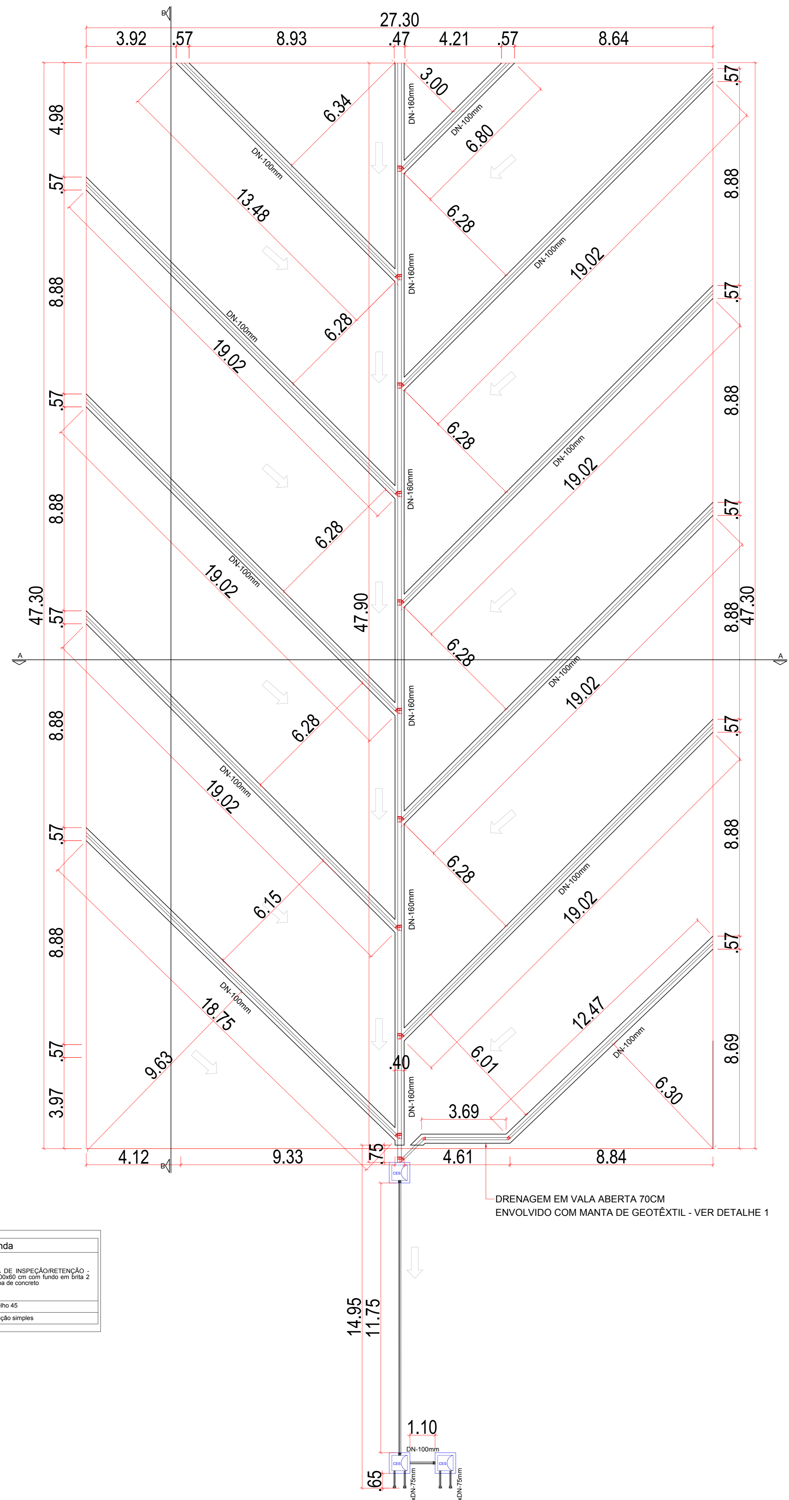
PLANTA BAIXA - DRENAGEM TIPO ESPINHA DE PEIXE Escala: 1/100
