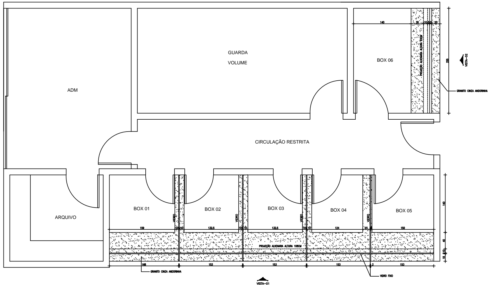
PLANTA ESCALA-1/25
