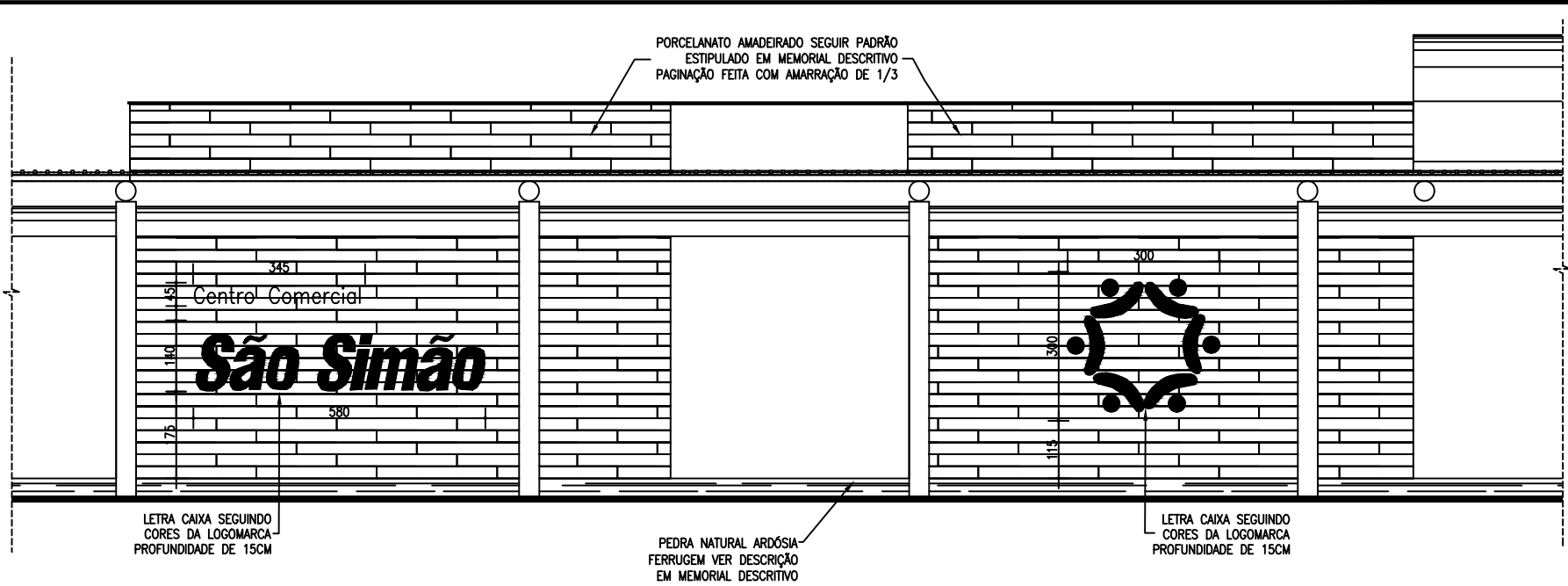
ELEVAÇÃO NOROESTE ESCALA-1/100
