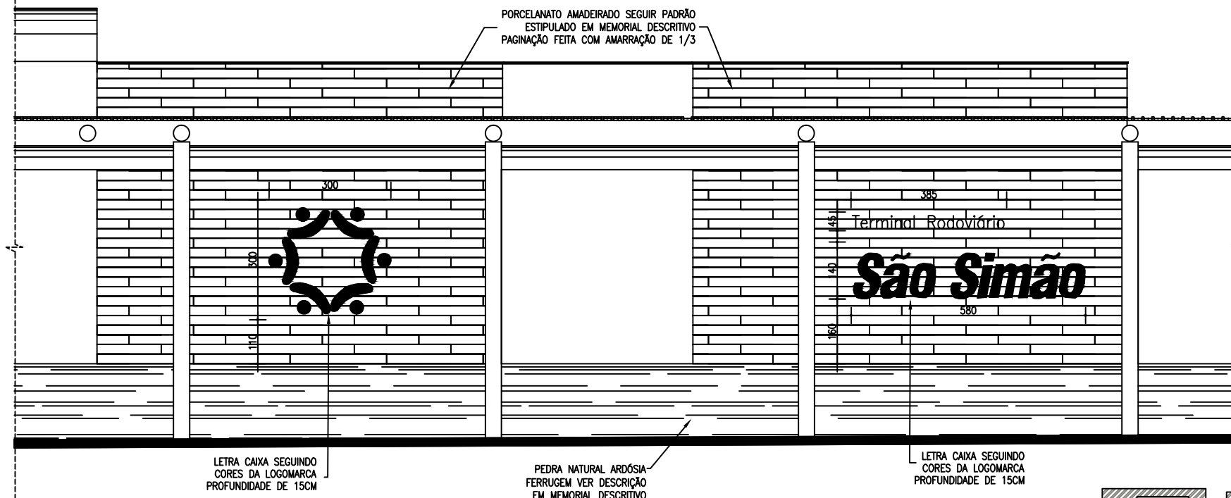
ELEVAÇÃO SUDESTE ESCALA-1/100
